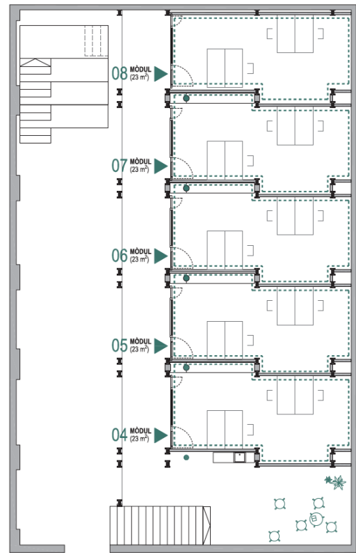
PLANTA ALTELL
