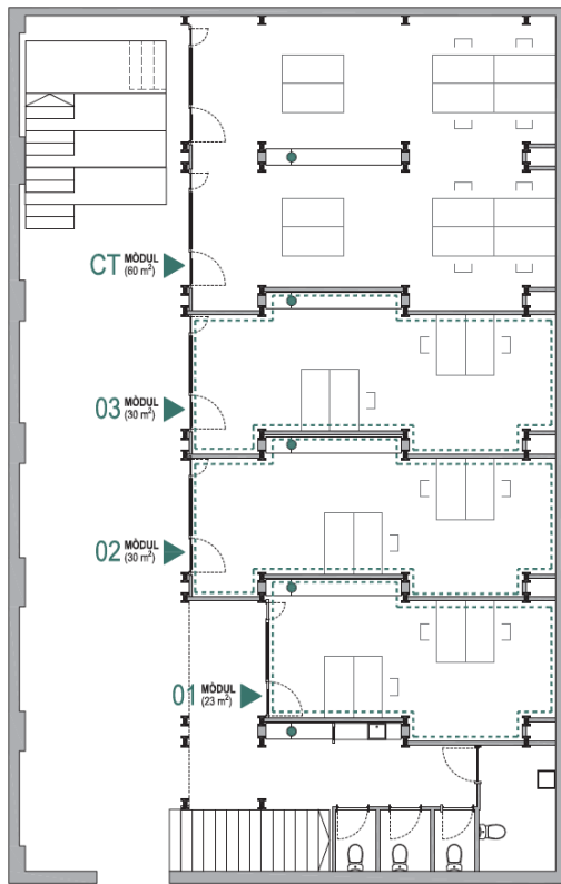
PLANTA BAIXA
